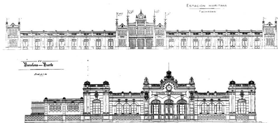
Figure 1.47 Drawings of Estacio Maritima and Embarcadero de Viajeros, Barcelona (Archivo Historico Puerto de Barcelona)
