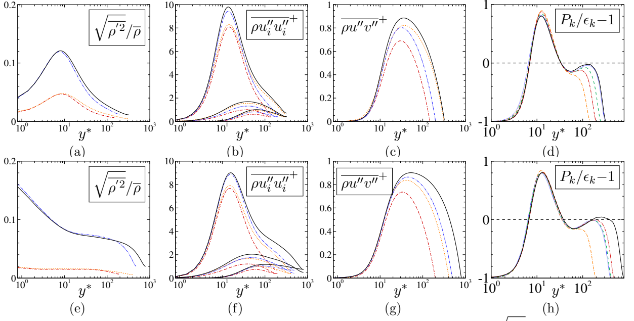
Figure 0.6. De gauche à droite: profils en y^* des fluctuations de densité ( \sqrt{\rho'^2}/\bar{\rho} ), tensions de Reynolds normales ( \overline{\rho u'' u''^+} ) et de cisaillement ( \overline{\rho u'' v''^+} ), et rapport production-dissipation de l'énergie cinétique turbulente ( P_k/\epsilon_k - 1 ). Ligne supérieure: air; ligne inférieure, PP11. Légende comme en tableau 0.2.
