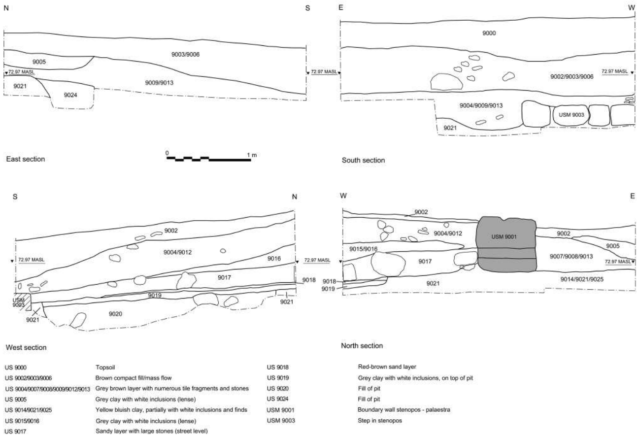
Fig. 18. Trench 9, sections (F. Spadaro, M. Trümper).
