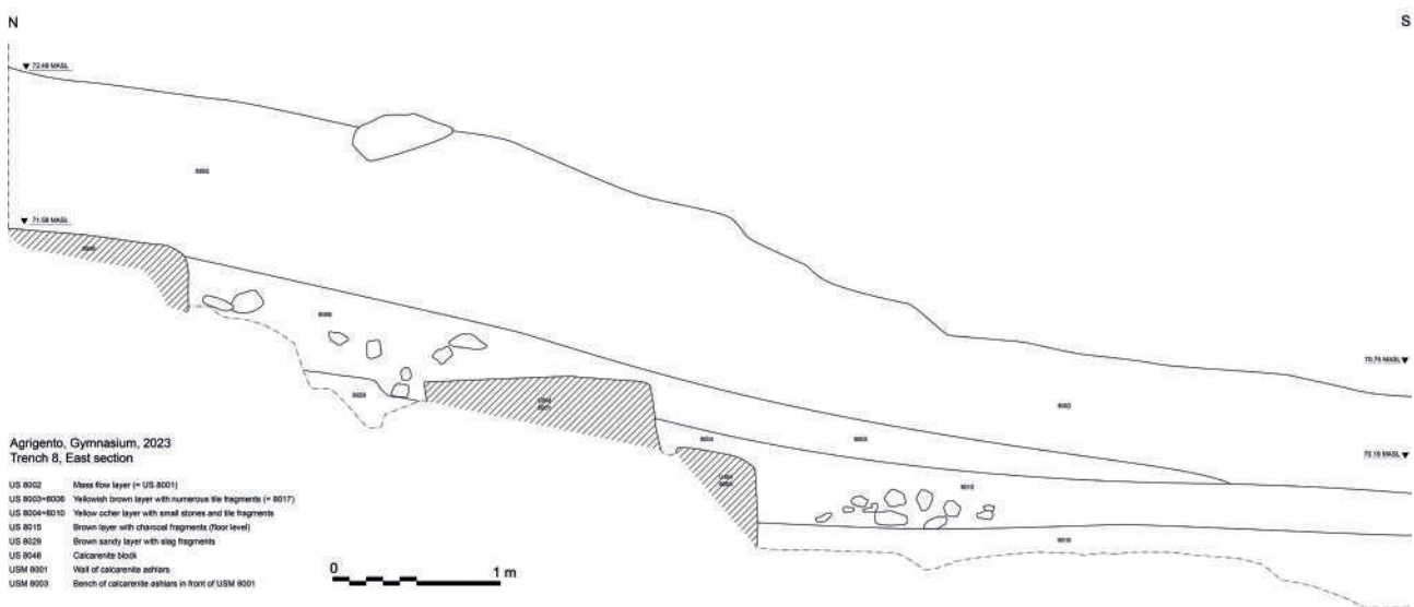
Fig. 5. Trench 8, east section (F. Birkner, T. Lappi).
