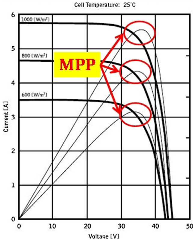
Fig. 6. MPPT plots.
