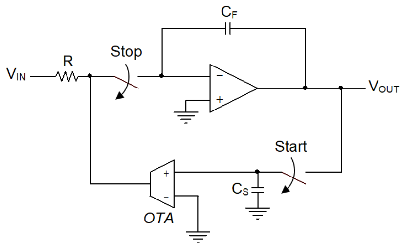
Fig. 21. Integrator of the ASIC PETA.
