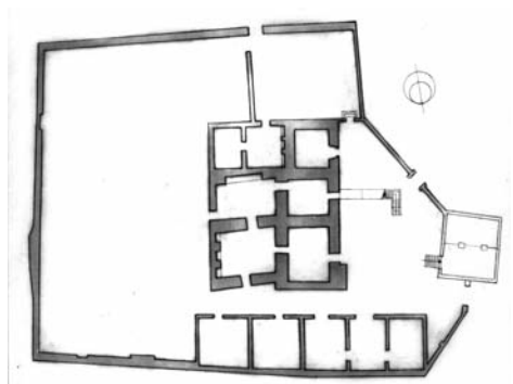
Figura 48: Masseria Cippano - Planimetria primo livello
