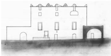
Figura 28: Masseria Musacco - Prospetto principale
