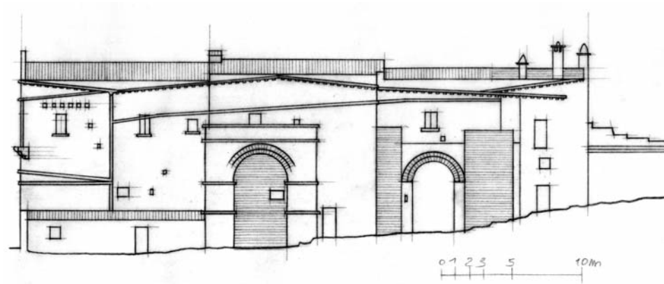
Figura 41 - 43: Masseria Jasca - Prospetti
