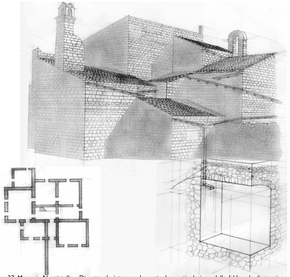
Figura 27: Masseria Nunziatella - Di notevole interesse la particolare articolazione delle falde e la diramazione assunta dalle linee di gronda per consentire all'acqua piovana di essere convogliata verso la cisterna
