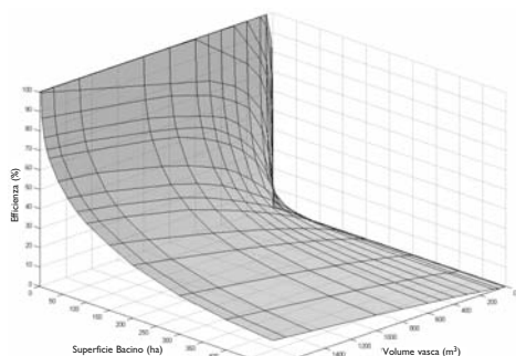
Figura 6: Andamento dell'efficienza per Ruvo di Puglia, anno 1997
