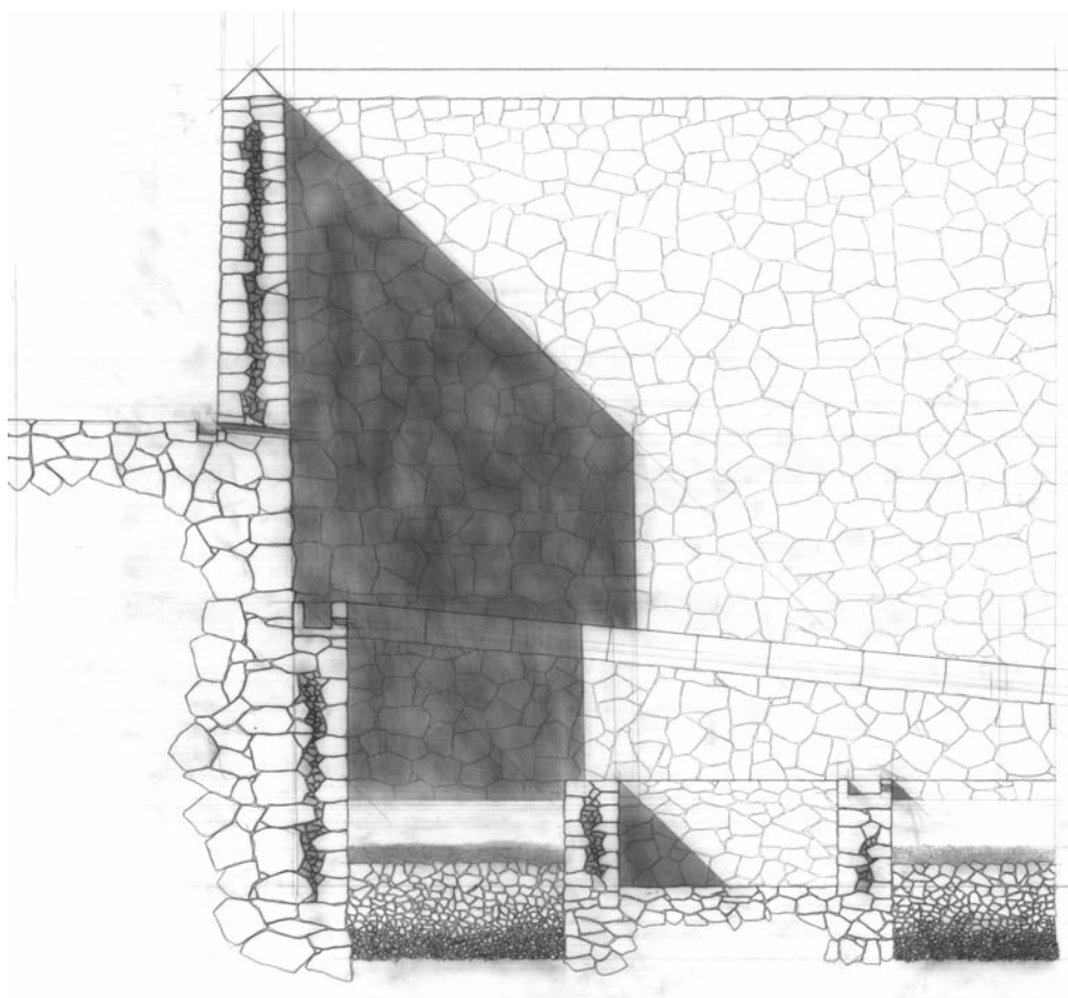
Figura 35: Masseria Losciale - Sistema di raccolta delle acque meteoriche nella piana coltivata ad agrumeto e vigneto.
