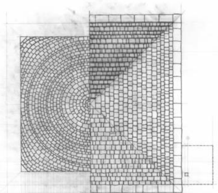
Figura 33: Masseria Cerere - Sezione e pianta della copertura della cisterna isolata
