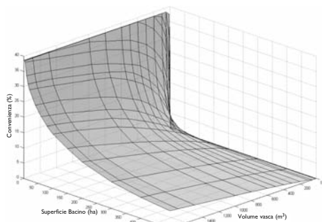
Figura 7: Andamento della convenienza per Ruvo di Puglia, anno 1997
