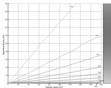
Figura 8: Abaco dell'efficienza per Ruvo di Puglia, anno 1997
