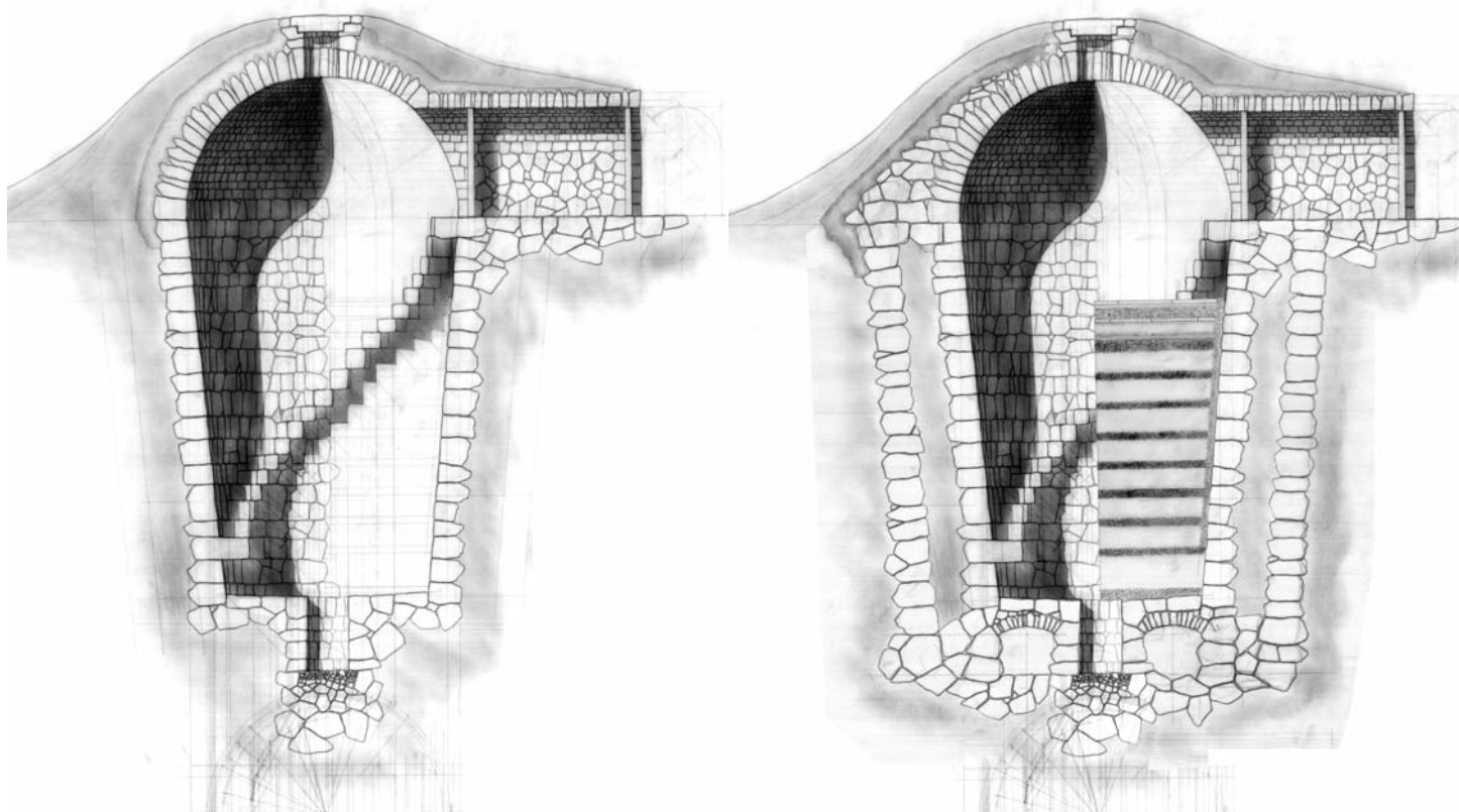
Figura 18 - 19: Schema di funzionamento di una neviaia ipogea e sue possibili varianti costruttive. Il secondo schema conserva i medesimi caratteri formali e funzionali del primo sistema architettonico ma evidenzia alcune differenze nel comportamento tecnico, tra cui, il potenziamento dell'isolamento dal terreno, attraverso l'impiego di un sistema murario a doppio paramento con camera d'aria, e l'introduzione di un piano di fondazione su vespajo che favorisce un più rapido smaltimento dell'acqua residuale, e incrementa l'isolamento rispetto all'umidità del terreno.
