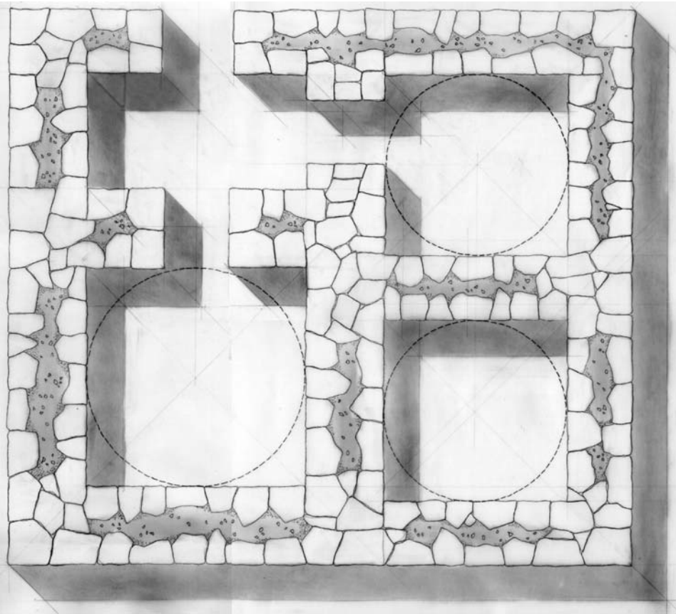
Figura 56: Planimetria esemplificativa di una struttura a trullo
