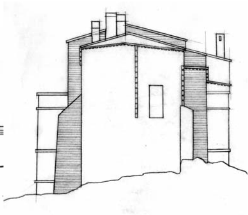
Figura 41 - 43: Masseria Jasca - Prospetti
