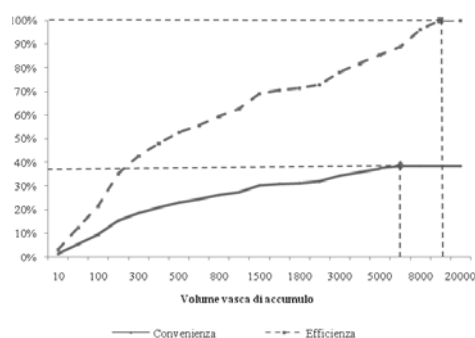
Figura 9: Andamento dell'efficienza e della convenienza per l'area di studio.
