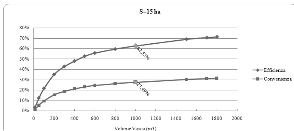
Figura 10: Andamenti di efficienza e convenienza al variare del volume per una superficie servita di 15 ha
