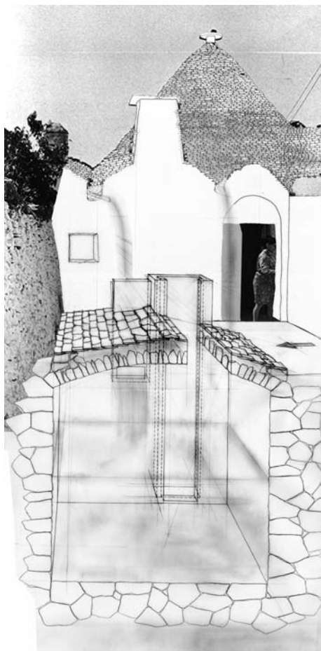
Figura 61 - 62: Esempi di cisterne urbane sotterranee in sistemi aggregati intorno ad una corte (sinistra) e lungo una strada (destra)
