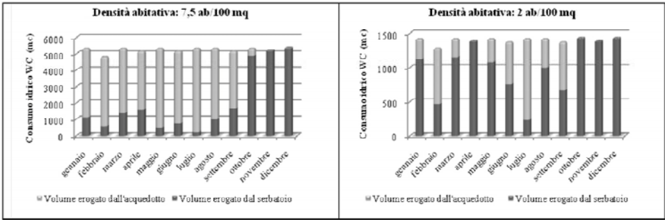
Figura 65: Confronto gradi di efficacia del sistema di accumulo e utilizzo delle acque meteoriche al variare della densità abitativa per Ruvo di Puglia.
