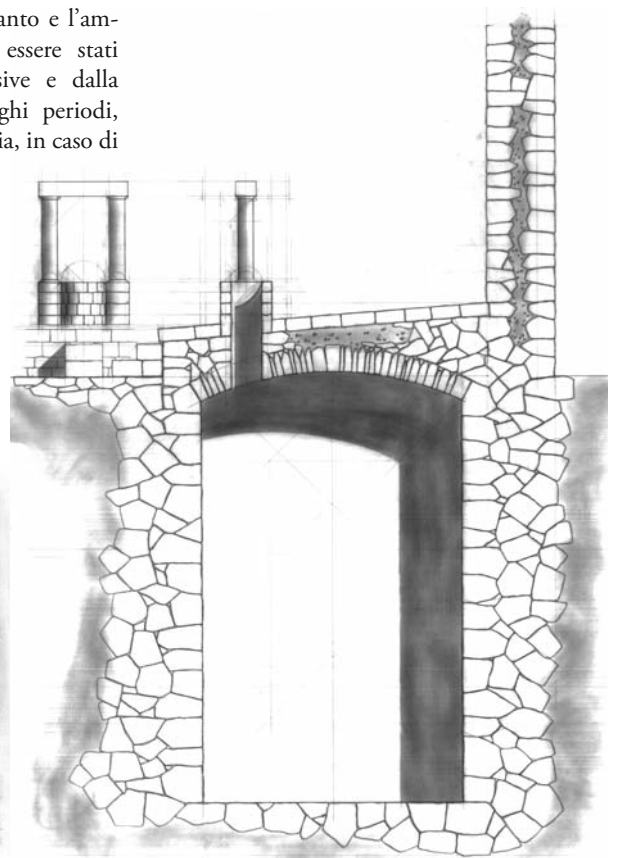
Figura 30: Masseria Musacco - Sezione della cisterna-pozzo
