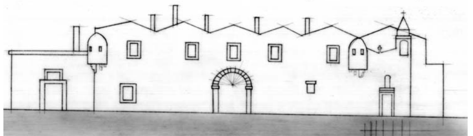
Figura 45 - 46: Masseria Viglione - Prospetto principale e laterale
