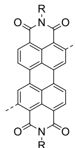
Perylenediimide
