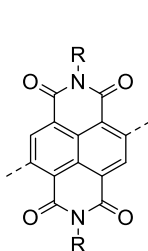
Naphthalenediimide
