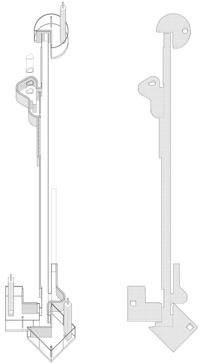
in questa pagina/ in this page: House 10: Assonometria monometrica / House 10: Monometric axonometry
